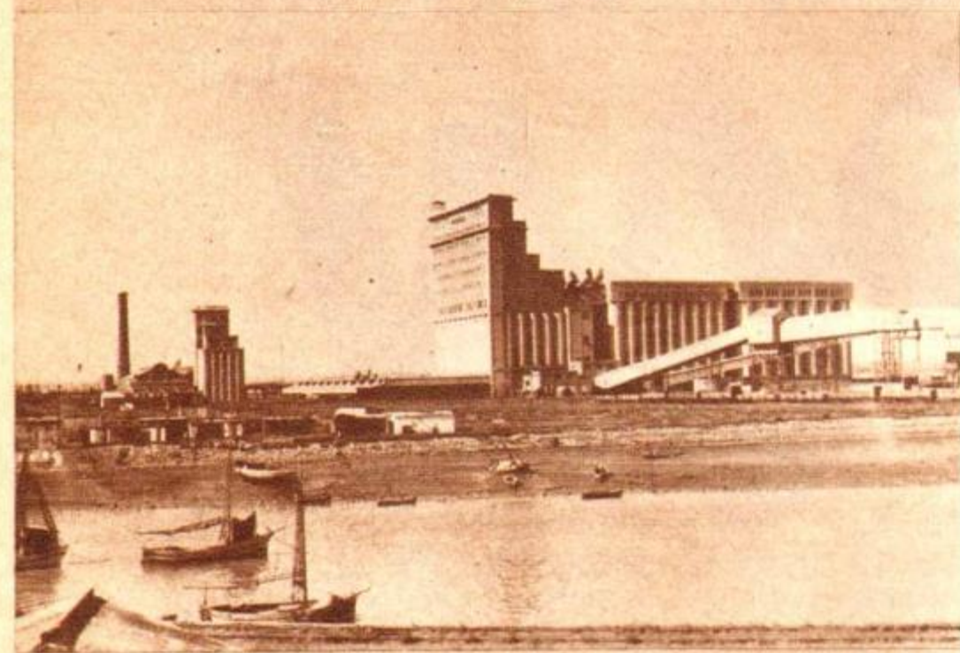
Elevador terminal de Ingeniero White, con capacidad para 142.000 toneladas, construido en Bahía Blanca.
